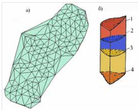
Рис. 1. Интегрированной пространственной модели рельефа, геологии и гидрогеологии местности: а) фрагмент триангуляции Делоне в плане в пределах полосы варьирования трассы; б) элемент пространственной триангуляции: 1 – земная поверхность, 2 – поверхность УГВ; 3, 4 – подошвы соответственно первого и второго слоев грунта
